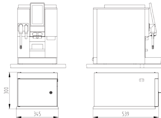
Unterstellkühlleinheit unter Kaffeemaschine
